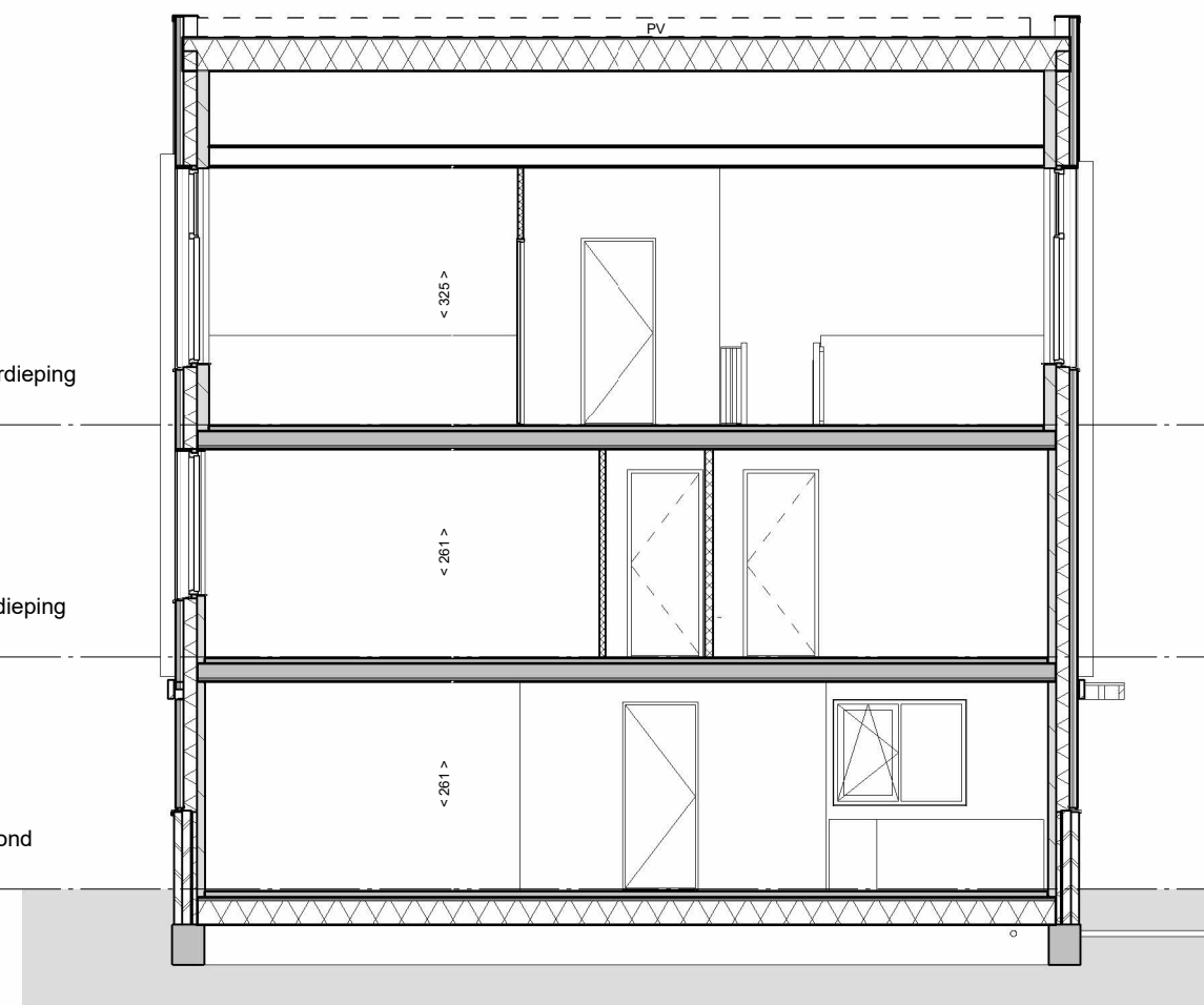
dwarsdoorsnede
