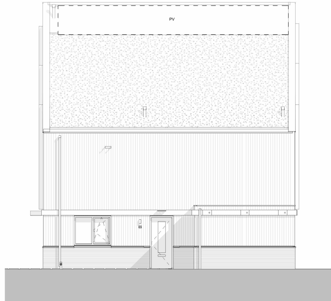
zijgevel (zuidoost)
